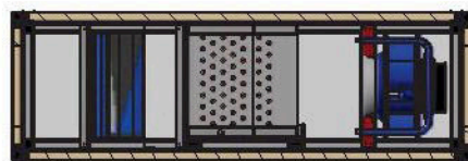
A-A ( 1 : 16 )
